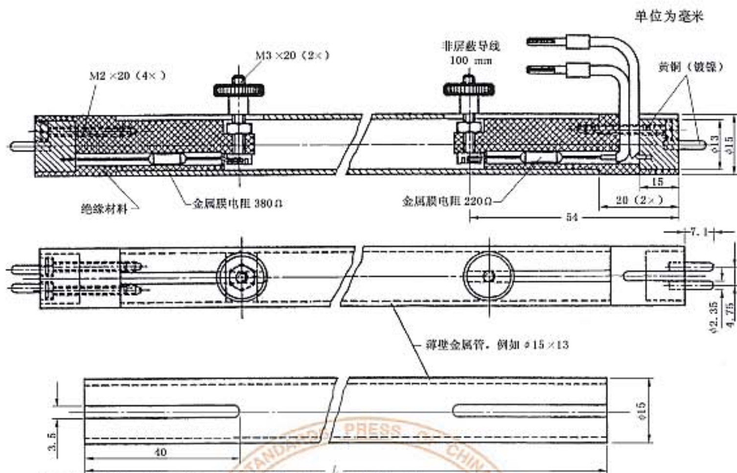
图 4c 15 mm 荧光灯的模拟灯
