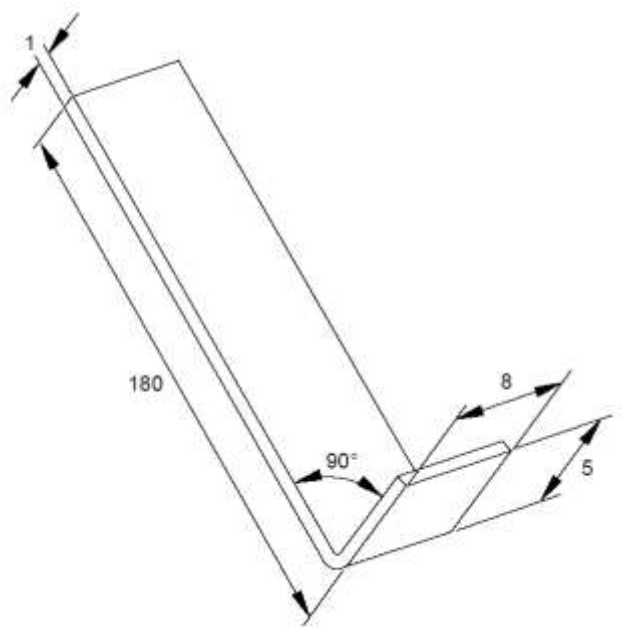
图4 试验钩
