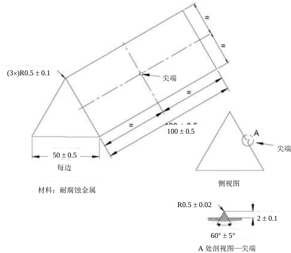
图14 芯轴
