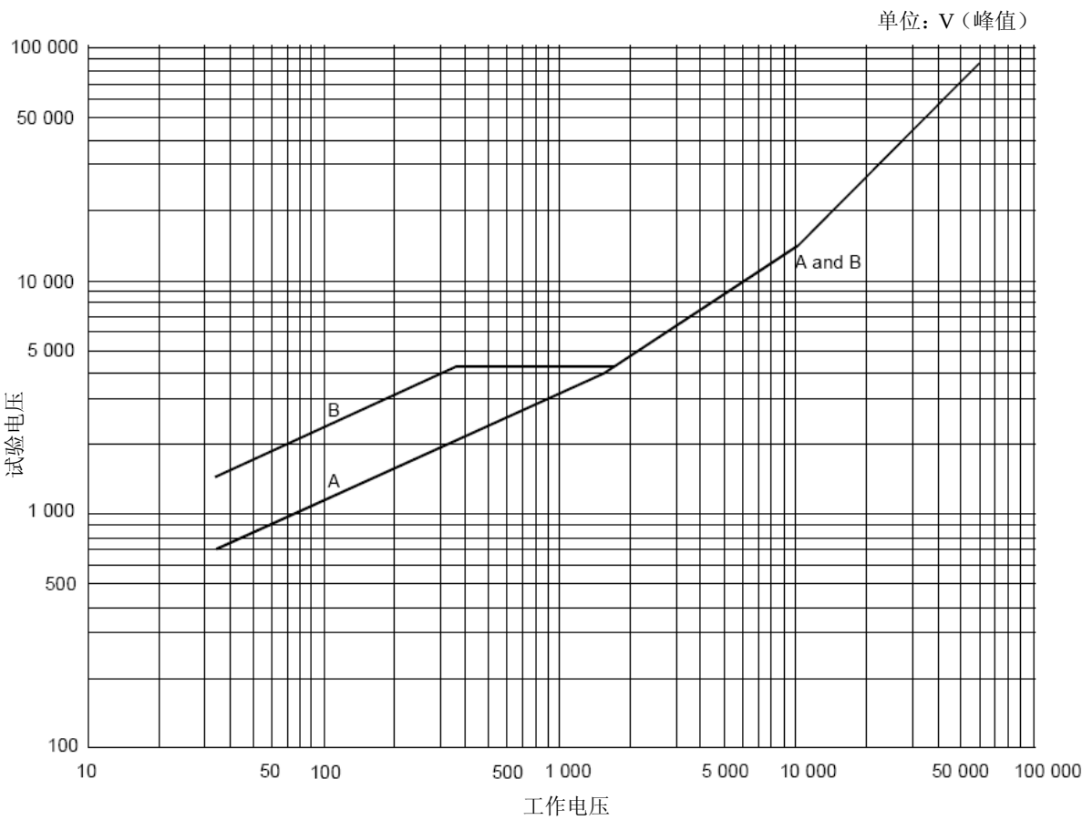
图7 试验电压
