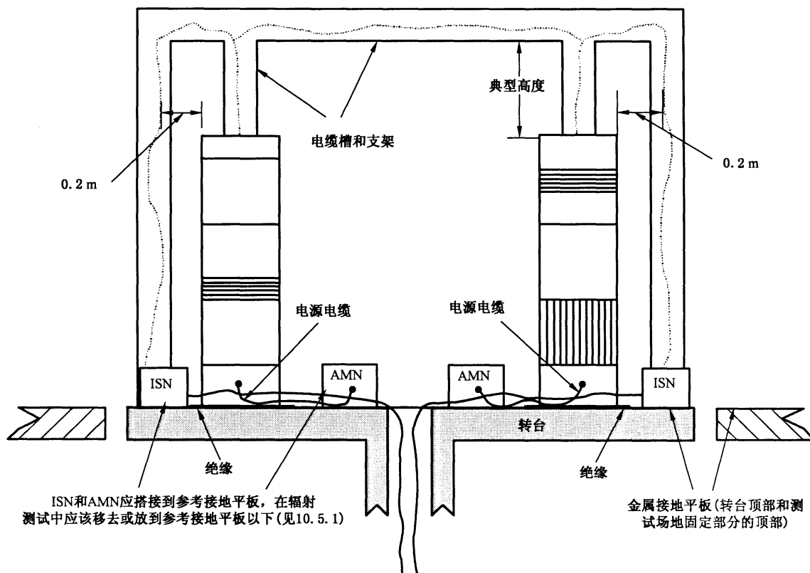
正视图
