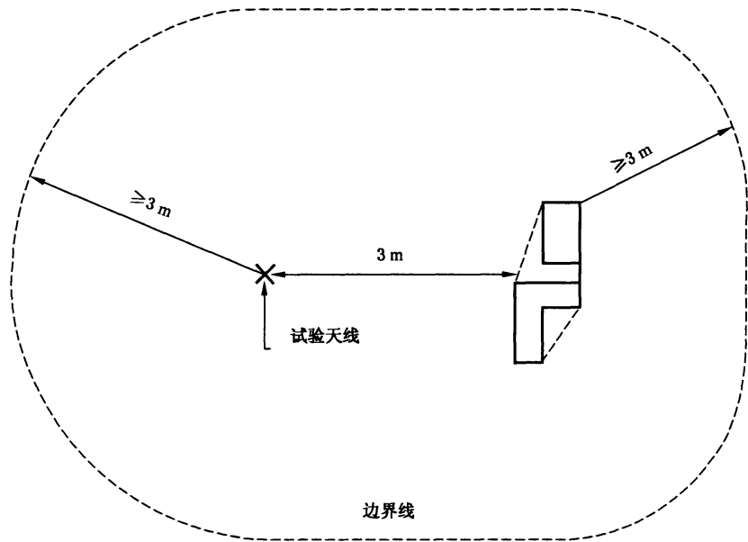
图形边界围绕的场地上方应无反射物。该空间的水平面高度相对于水平接地平板应至少比天线与受试设备之最高点高 3 m。 注：替换场地的适用性见 10.4.3, 场地边界的确定方法见 10.3.1。
