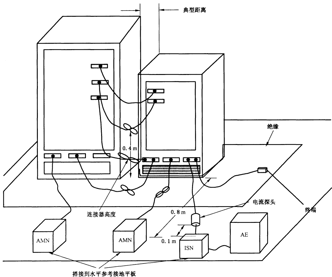
图 8 落地式设备测试布置示意图(传导发射测量)
