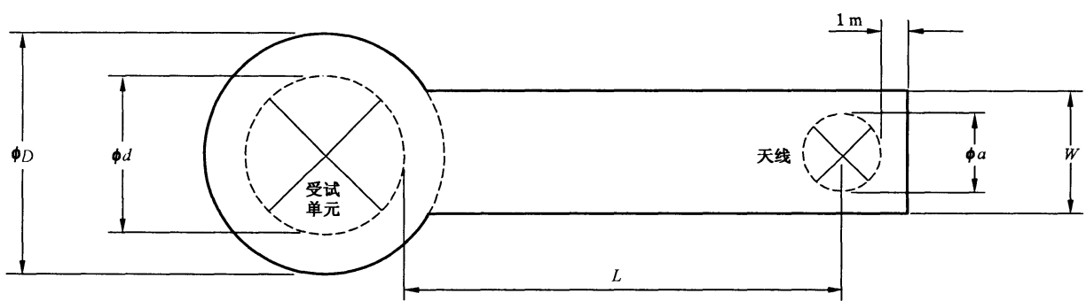
D=d+2\text{ m} , 其中 d 为 EUT 的最大外径; W=a+2\text{ m} , 其中 a 为天线的最大外径; L=3\text{ m} 或 10\text{ m} 。
